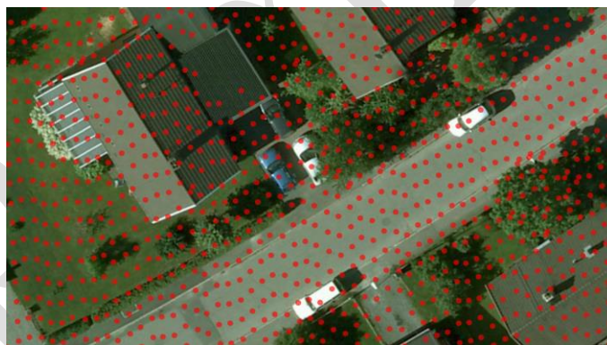
Figur 2.3.2.b Exempel på träffbild med låg punkttäthet. I vegetation ökar tätheten eftersom varje utsänd laserpuls där kan ge flera returer på olika höjd. Notera att ett hustak saknar punkter.
