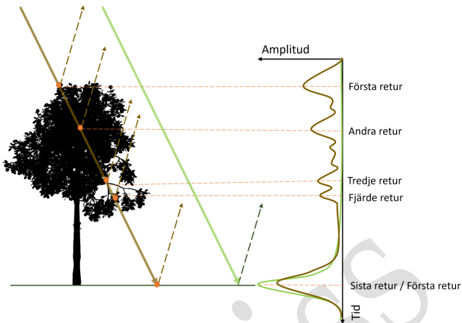
Figur 2.3.2.a Punkttätheten ökar i skog eftersom varje utsänd puls där kan ge flera returer. På öppen mark kan en utsänd puls endast ge en retur.
