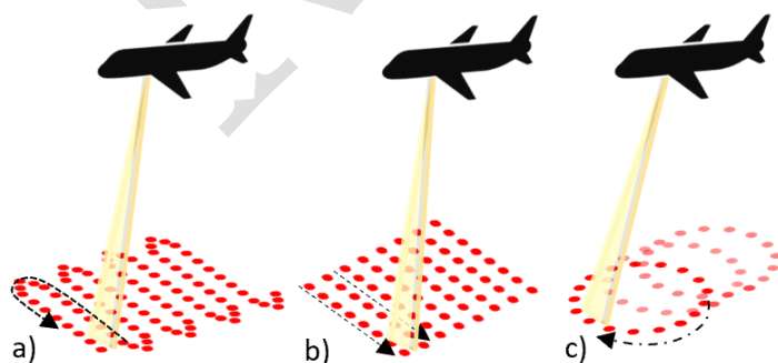
Figur 2.3.2.c Punkt a-c illustrerar tre vanliga skanningsmönster hos flygburna lasersensorer: a) Oscillerande b) Linjärt c) Cirkulärt (Palmer).
